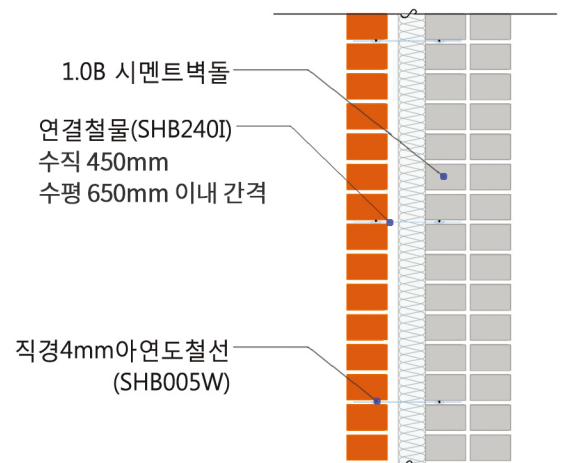
단면도
