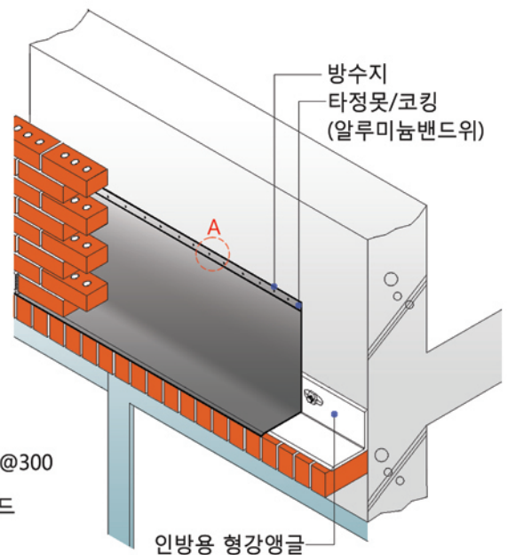
개구부 상부(앵글상부)
